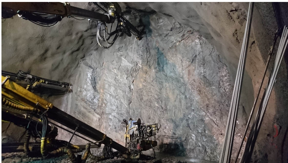
Figur 12 I stoffen ved pel nr. 13302 oppsto det jekking
