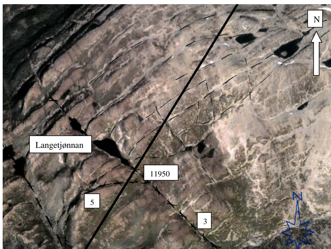
Figur 19 Tolkning av strukturegeologien i området, (tykk svart strek er tunneltraseen).
