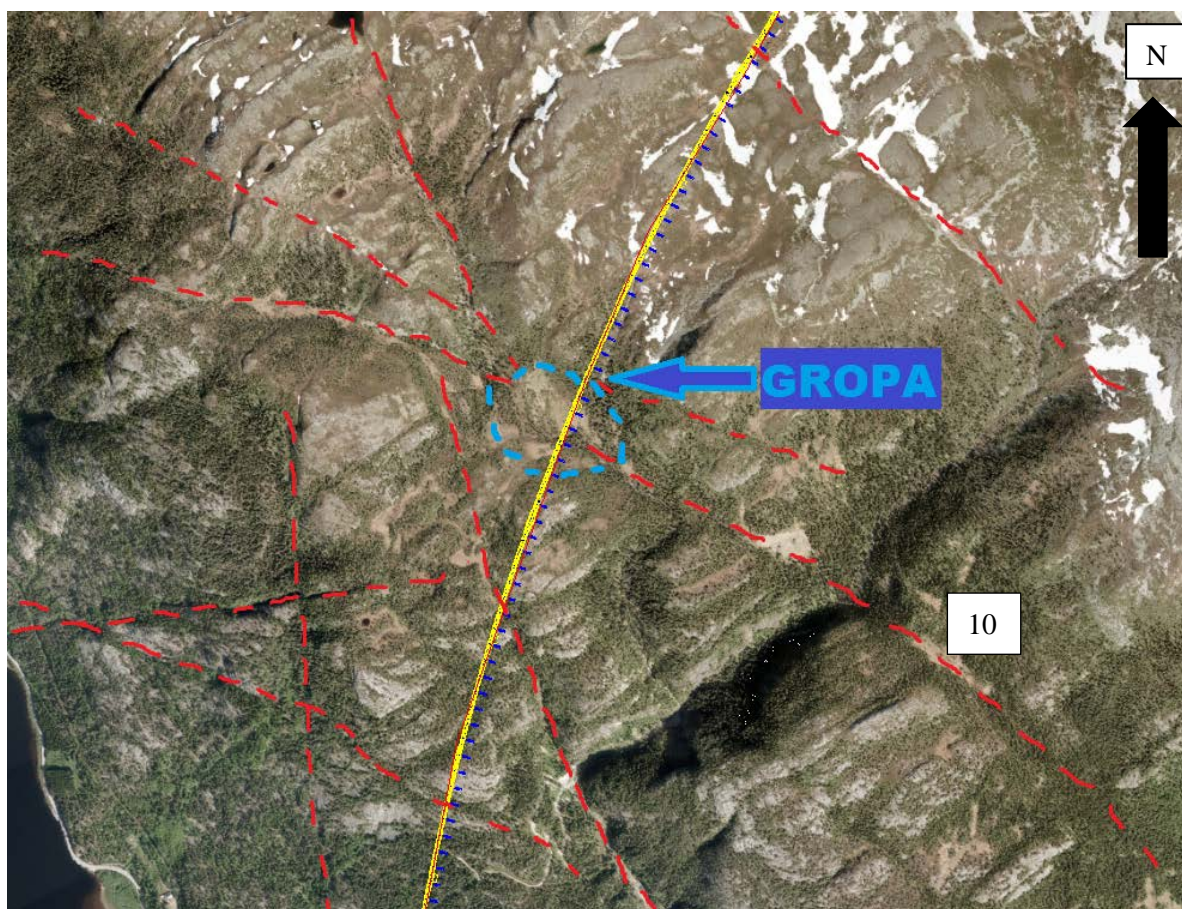
Figur 5 Struktureologisk tegning fra SVV
