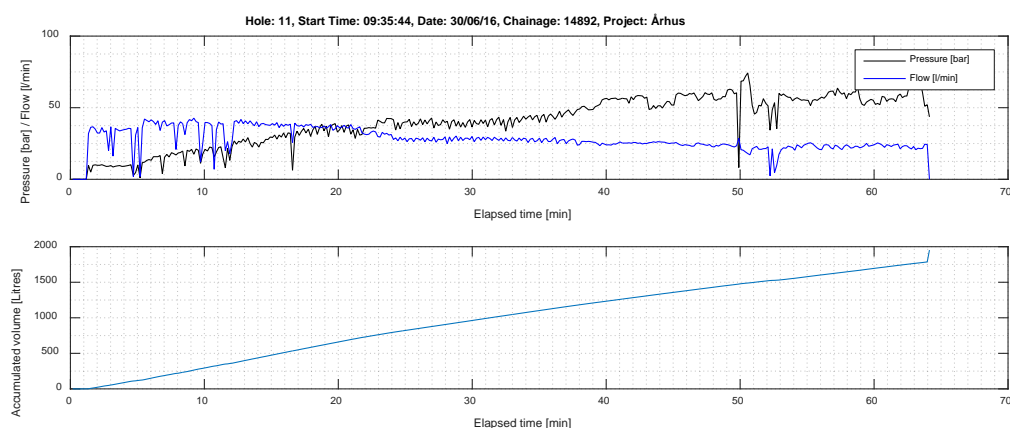
Figur 23 Eksempel fra borhull 11 i skjerm ved pel nr. 14892
