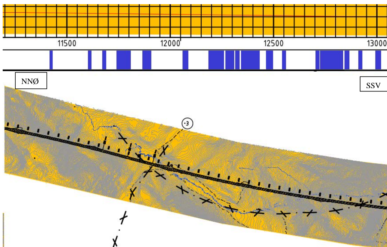
Figur 20 Lengdeprofilen øverst viser strekninger med injeksjon (blått) og nederst vises ingeniørgeologisk kart med inntegnede svakhetssoner (Sweco, 2014)
