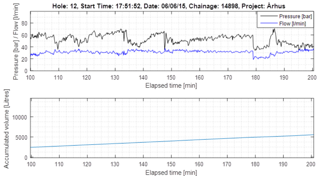
Figur 22 Eksempel på jekking i borhull 12
