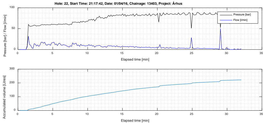
Figur 24 Eksempel fra borhull 22 i skjerm ved pel nr. 13403
