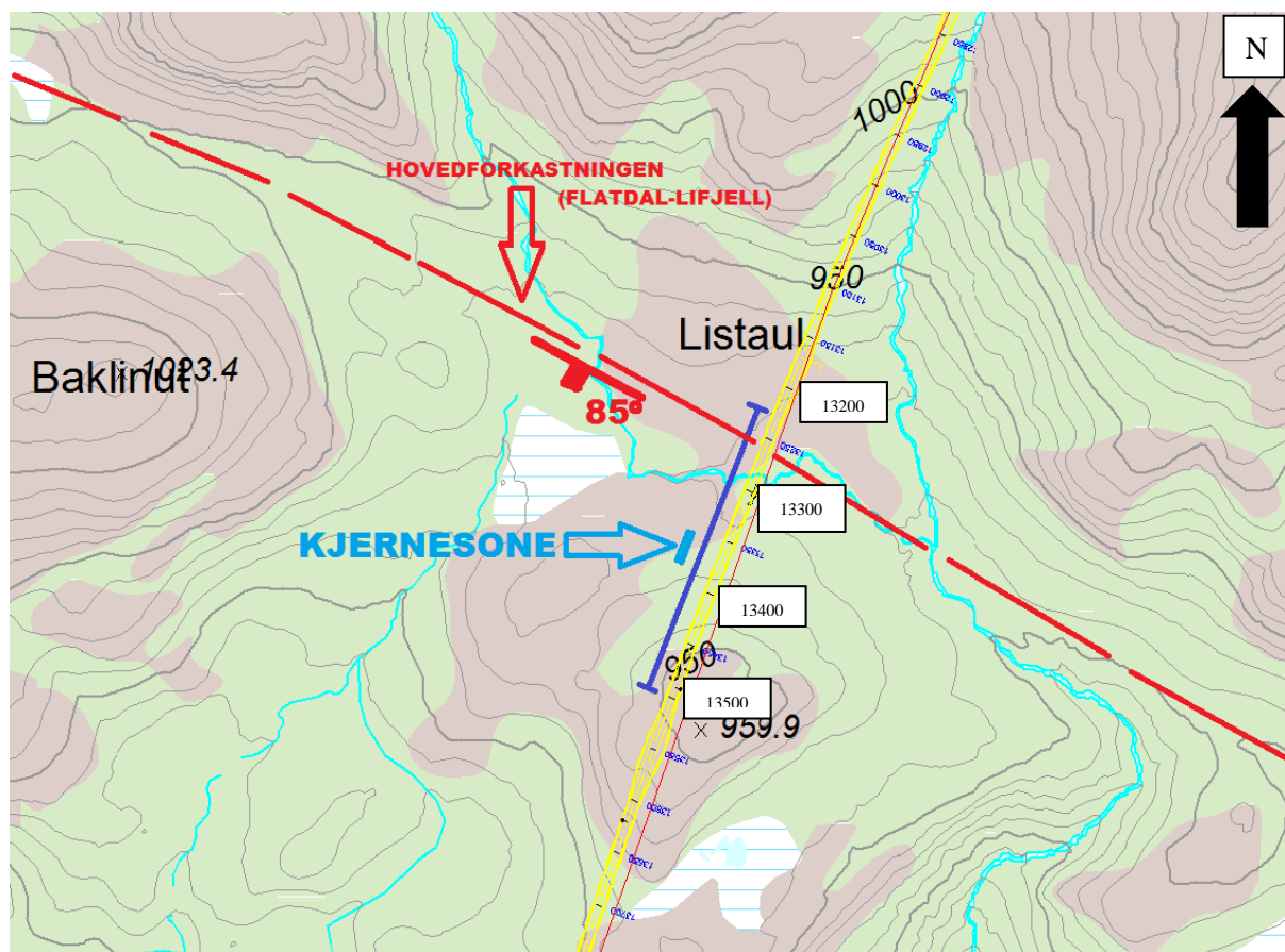
Figur 6 Strukturgeologisk og topografisk tegning over sonen, SVV
