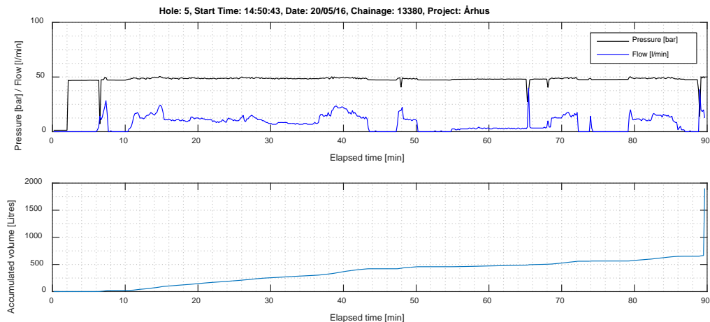
Figur 25 Eksempel fra borhull 5 i skjerm ved pel nr. 13380
