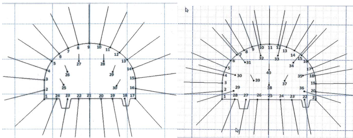
Figur 9 Injeksjonsskjerm; Sonder 1 til venstre og sonder 2 til høyre
